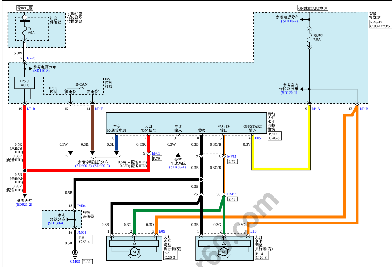
自动大灯水平调整系统(AHLS)(1)
